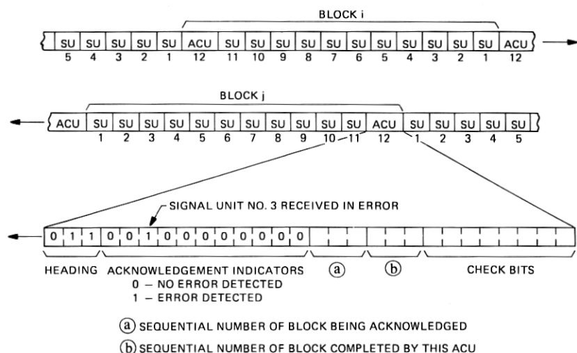
Fig. 5—Block structure, CCIS SUs and ACU.
